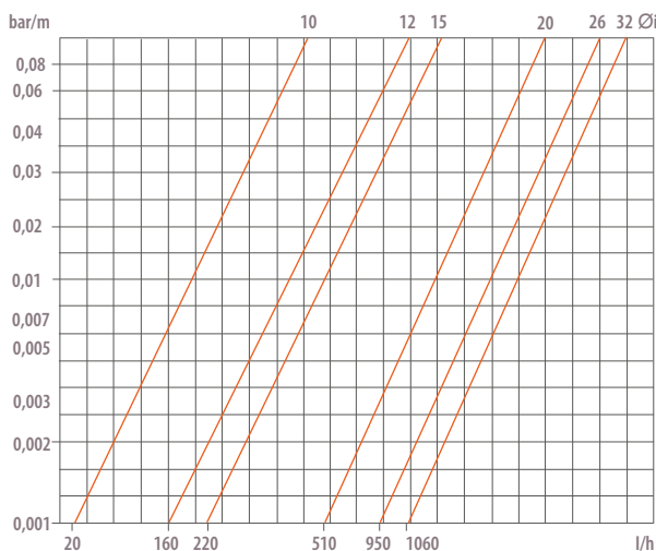
Caduta di pressione per metro di tubo in lunghezza rettilinea
