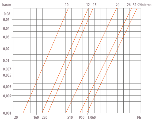
Caduta di pressione su entrambi i raccordi dritti
